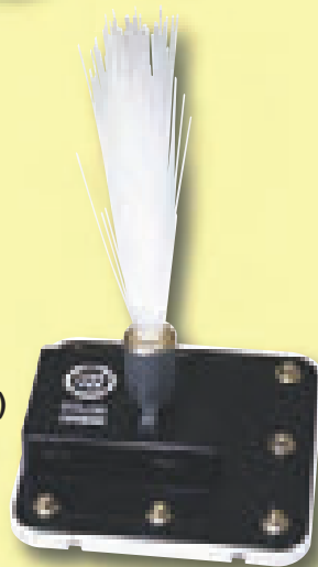
Rozvětvený optický kabel (LED doplněk) zapojen do U22
