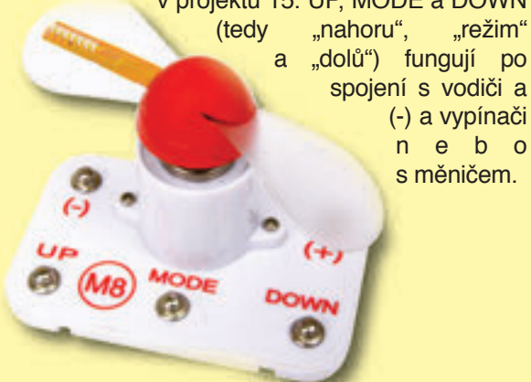
Programovatelný větrák (M8)
